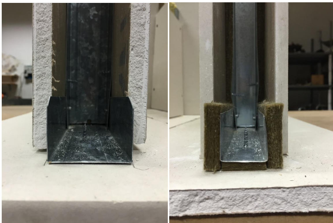
Senza correzione termoacustica
